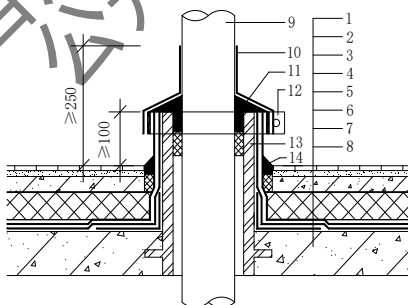
1—屋面饰面层；2—细石混凝土保护层；3—隔离层；4—保温层；5—防水层 1；6—防水层 2； 7—管根节点防水；8—屋面混凝土结构；9—管道；10—高分子防水涂料； 11—高分子密封胶；12—金属箍；13—预埋套管；14—密封胶
