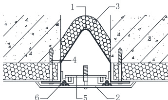
1—三元乙丙止水带；2—金属面板；3—镀锌钢板-聚乙烯复合板；4—膨胀螺栓；5—不锈钢滑杆；6—橡胶止水条
