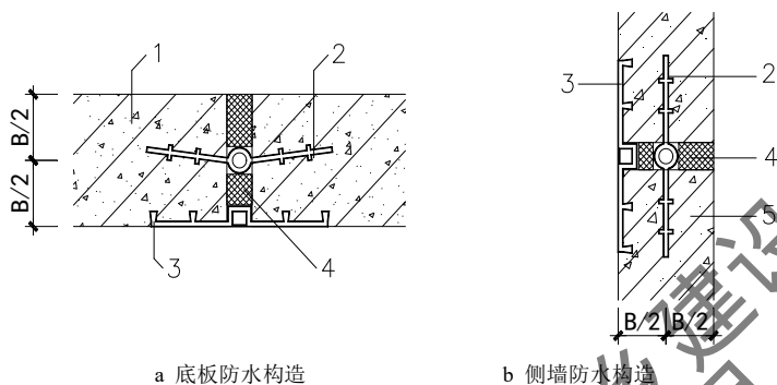
1-混凝土结构底板；2-中埋式止水带；3-外贴式止水带；4-衬垫板；5-混凝土结构侧墙
