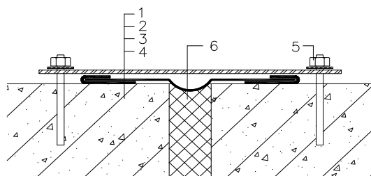
1—金属板压置；2—胶粘性止水带；3—胶粘剂；4—混凝土结构；5—膨胀螺栓； 6—变形缝模板
