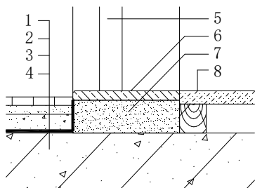
1—地面砖及粘结层；2—细石混凝土或砂浆保护层；3—防水层；4—混凝土楼板；5—门框； 6—门槛石；7—聚合物水泥防水砂浆挡水坎；8—干区地面饰面层
