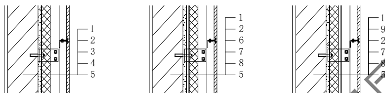
a 普通防水砂浆找平+聚合物水泥防水砂浆或防水涂料构造做法
