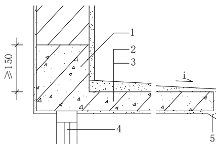
1—雨篷梁；2—聚合物水泥防水砂浆找坡；3—混凝土雨篷板；4—门窗；5—滴水线
