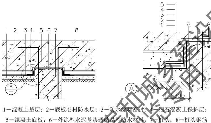
图 4.2.35 底板防水层为防水卷材的桩头防水构造
