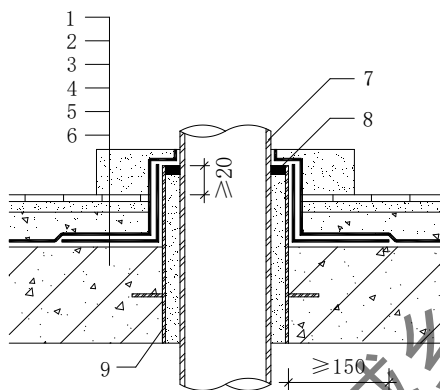
1—水泥砂浆护台；2—地面砖；3—细石混凝土保护层；4—防水层；5—套管根部节点防水； 6—混凝土结构楼板；7—穿楼板管道；8—高分子密封胶；9—预埋止水套管
