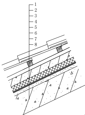
1—块瓦；2—挂瓦条；3—顺水条；4—细石混凝土持钉层；5—保温层； 6—防水层或防水垫层；7—水泥砂浆找平层；8—混凝土屋面板
