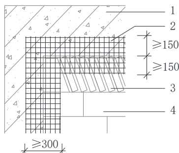
1—混凝土框架梁；2—玻纤网格布；3—斜砖顶砌；4—砌体墙
