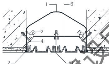
1—三元乙丙止水带；2—密封胶；3—弹性橡胶面板；4—膨胀螺栓；5—铝合金基座；6—不锈钢滑杆
