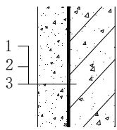
1—支护结构；2—预铺反粘防水卷材或预铺反粘卷材+其他防水卷材； 3—地下室混凝土侧墙
