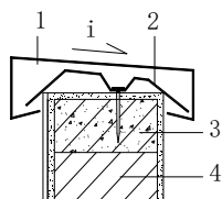
1—金属板压顶；2—固定支架；3—混凝土连梁；4—砌体女儿墙
