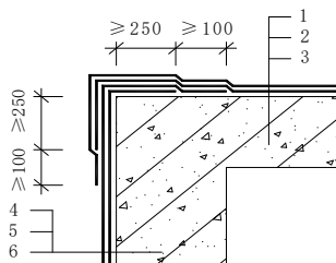
a 外设2道防水层搭接
