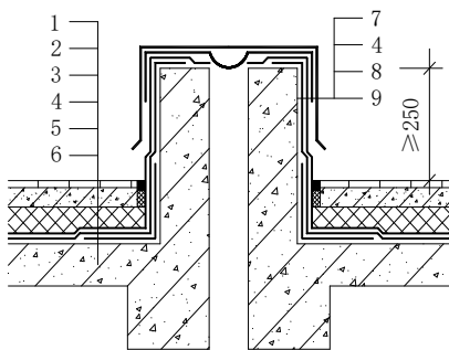
1—屋面饰面层；2—细石混凝土保护层；3—保温层；4—屋面防水层；5—阴角节点防水层； 6—屋面混凝土结构；7—现浇混凝土挡墙；8—塑料类防水卷材盖条；9—金属盖板
