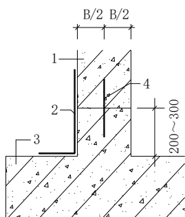
a 底板外挑结构、钢板止水带或自粘丁基橡胶钢板止水带
