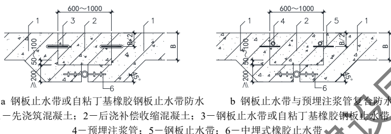
图 4.2.32-2 超前止水后浇带底板防水构造
