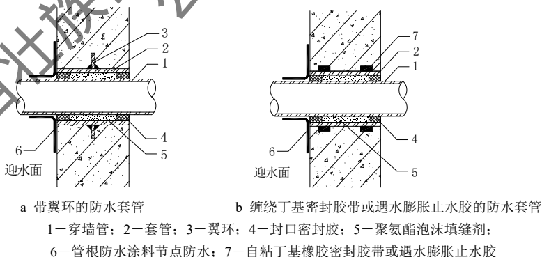
图 4.2.33 预埋套管穿墙管防水构造
