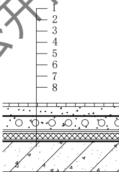
1—地面砖及粘结层；2—细石混凝土；3—高分子涂料防水层； 4—水暖盘管细石混凝土埋置；5—真空镀铝聚酯膜；6—XPS 保温板； 7—高分子涂料防水层或防水砂浆+高分子涂料防水层；8—混凝土结构楼板
