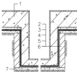
1—结构底板；2—内防水层；3—现浇混凝土坑、槽壁；4—外防水层；5—水泥砂浆找平层；6—砖胎模；7—混凝土垫层
