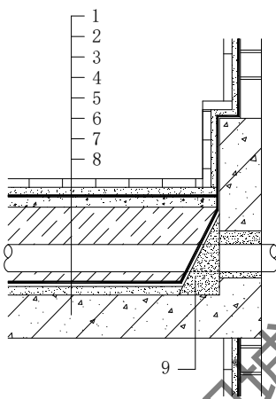
1—地面砖及粘结层；2—保护层；3—防水层 1；4—找平层；5—回填层涂料防水层； 6—管道；7—防水层 2；8—现浇混凝土结构楼板；9—混凝土或砂浆封堵
