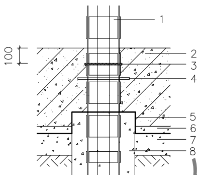
1—钢格构柱；2—混凝土结构底板；3—遇水膨胀止水胶；4—止水钢板； 5—桩头及底板防水层；6—细石混凝土保护层；7—混凝土垫层及找平层； 8—混凝土搅拌桩
