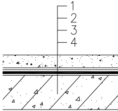
1—混凝土保护层；2—隔离层；3—防水层（1道或2道）；4—防水混凝土顶板
